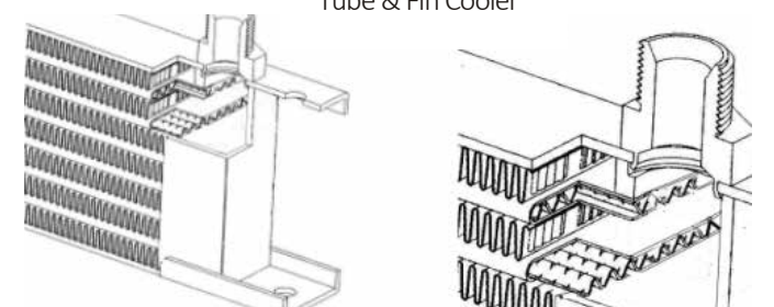
Tube & Fin Cooler
